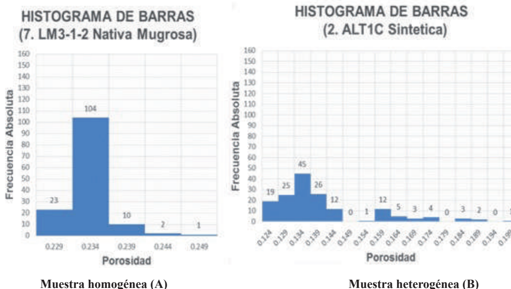
FIGURA 10. Histogramas de barras de la muestra 7 muestra homogénea A , y la muestra B que es heterogénea, se nota la variación de porosidad en la muestra 2. ALT1C Sintética por tener muchos intervalos del eje X y así mismo los datos están muy repartidos en cada uno de esos intervalos, en cambio la muestra homogénea tiene pocos intervalos y tiene un alto porcentaje de datos en un solo intervalo.
