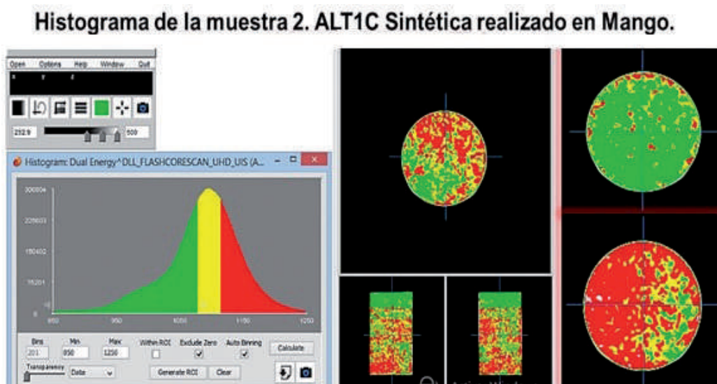
FIGURA 12. Visualización con el software Mango de histograma de la muestra 2. ALT1C Sintética.
